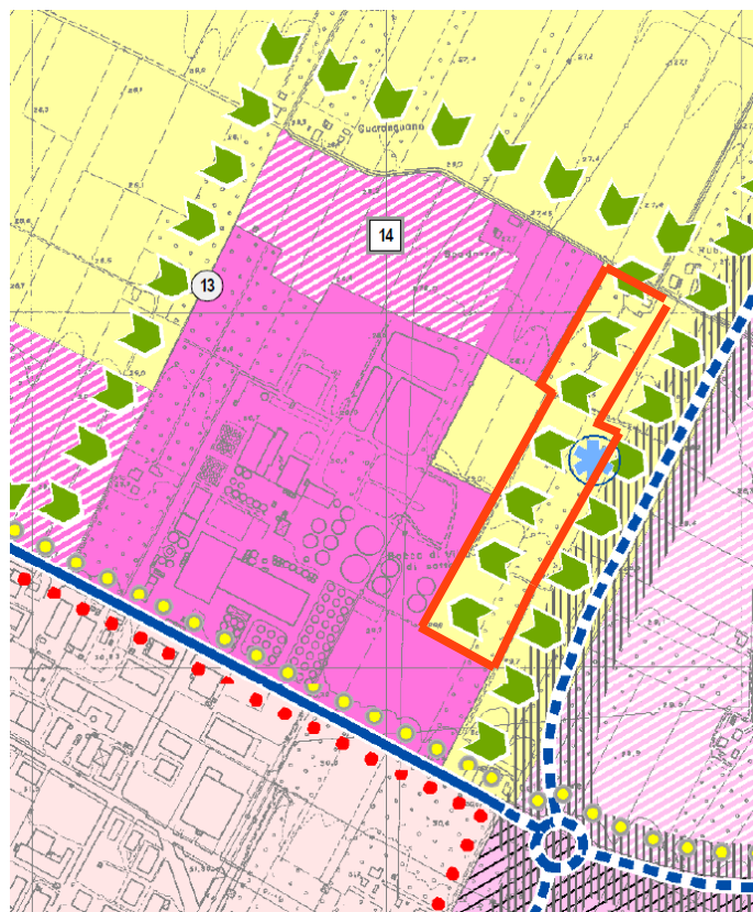
Figura 6: Stralcio PSC
