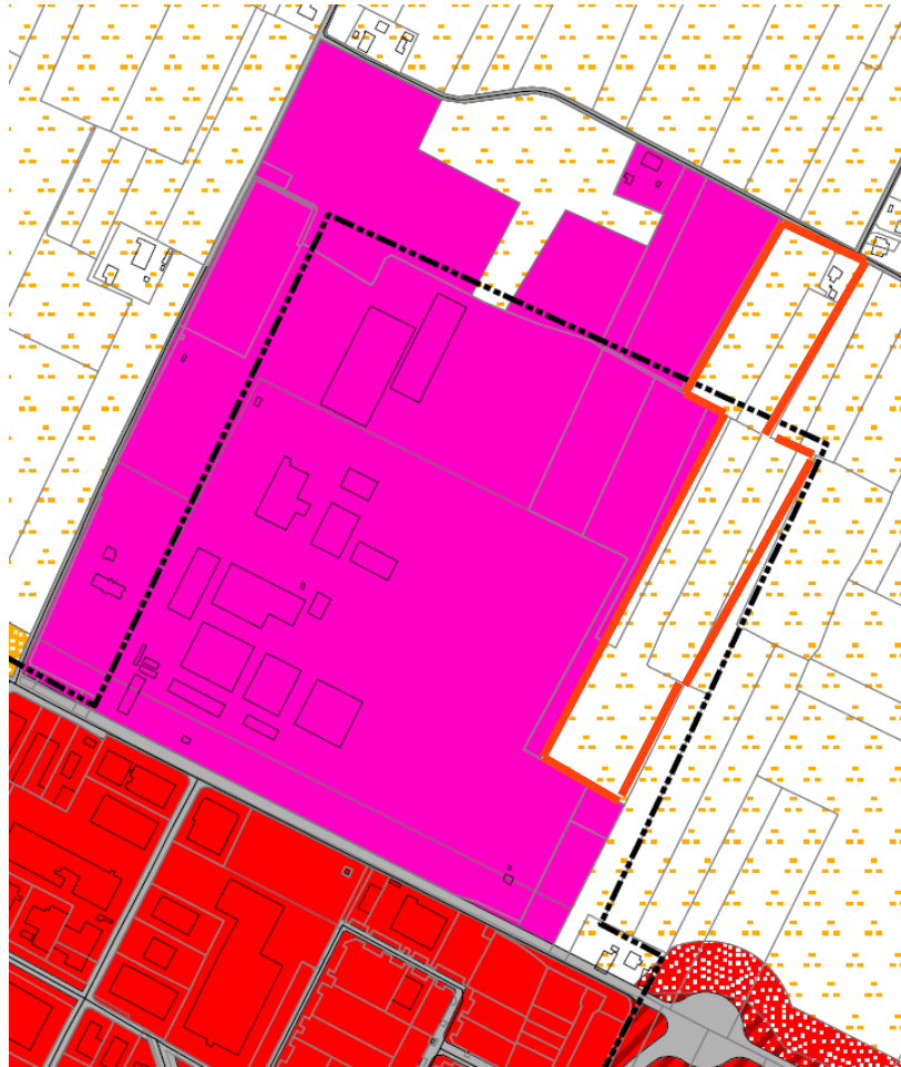
Figura 8: Stralcio PCA
